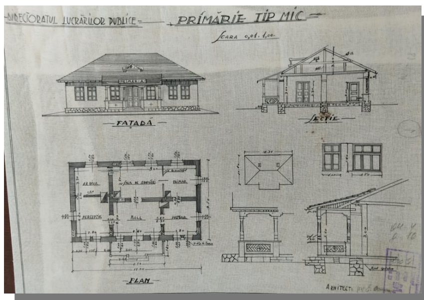
Figura 23. Plan de edificare a primăriei de tip mic. Sursă: ANA, F. 11, inv. 4, d. 16, f. 1.
