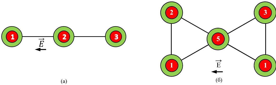
Рис. 1. Геометрические конфигурации тримера (а) и пентамера (б).
